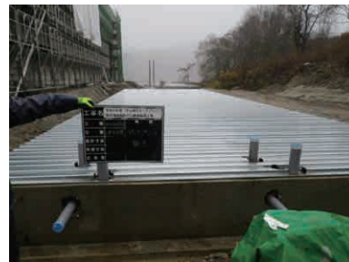
土壌浸潤槽 デッキプレート完成(埋戻し前)
